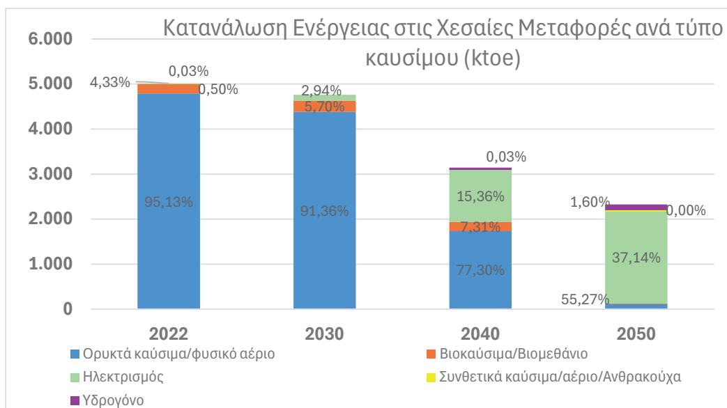
Σχήμα-ΕΣ 15 Κατανάλωση ενέργειας στις χερσαίες μεταφορές ανά τύπο καυσίμου (κτοε).
