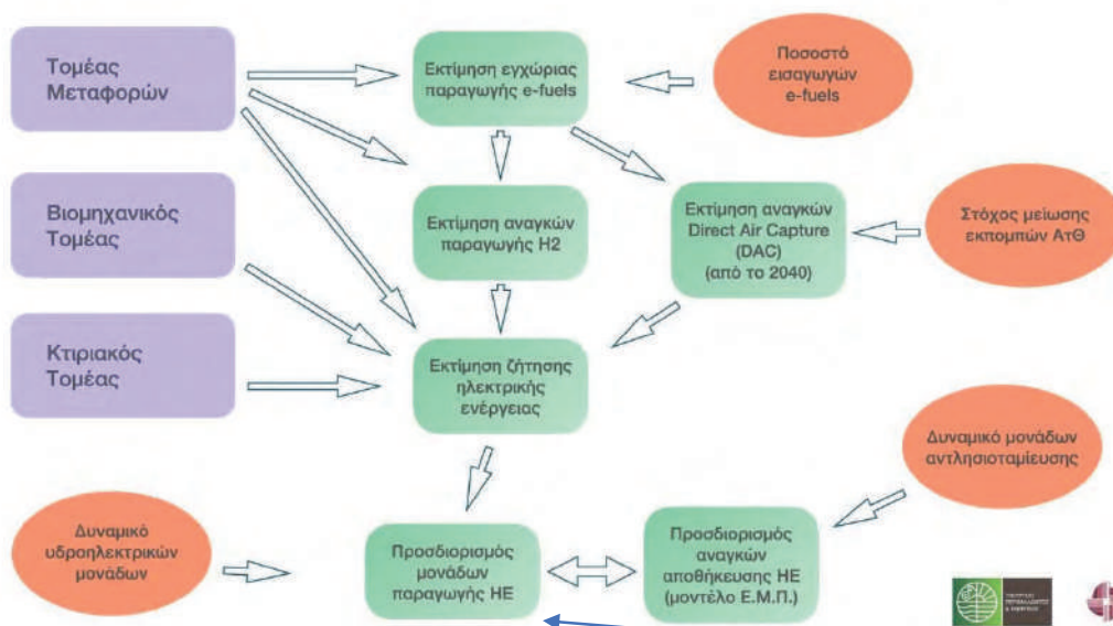
Σχήμα-ΕΣ 4 Σχηματική παρουσίαση ροής υπολογισμών προσδιορισμού μονάδων ηλεκτροπαραγωγής και αποθήκευσης ενέργειας.
